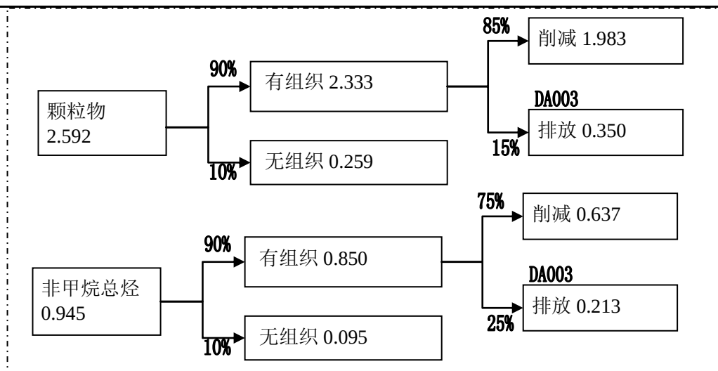
图 4.2-2 喷漆、烘干固化废气物料平衡图 (单位: t/a)
