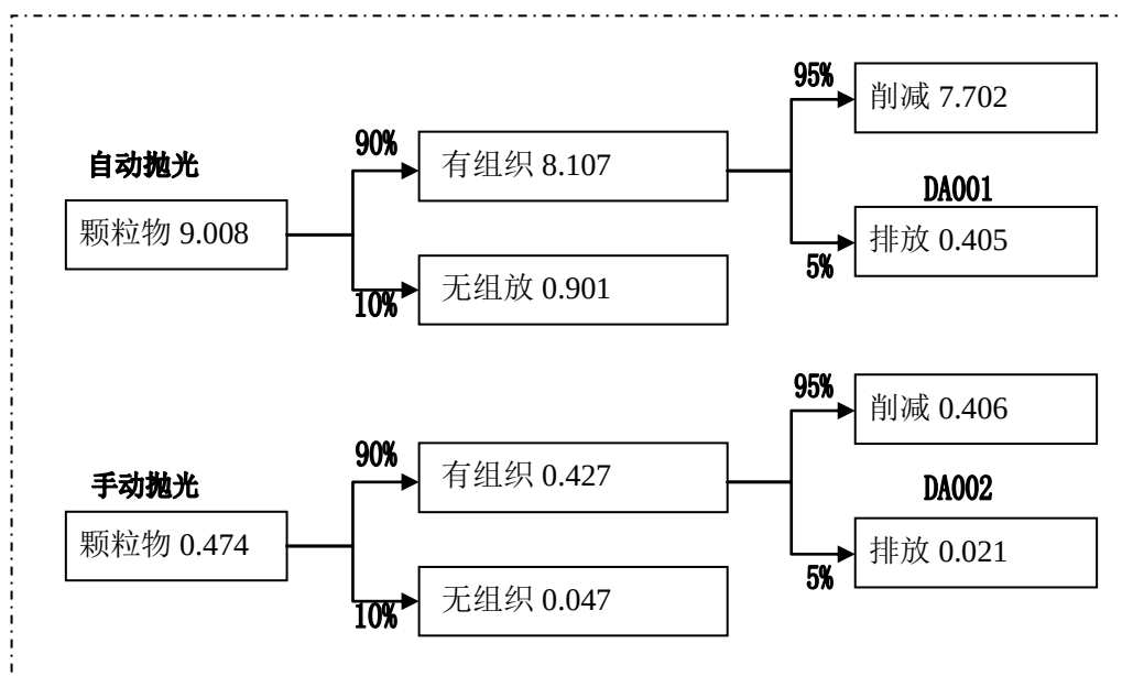
图 4.2-1 抛光粉尘物料平衡图（单位：t/a）
