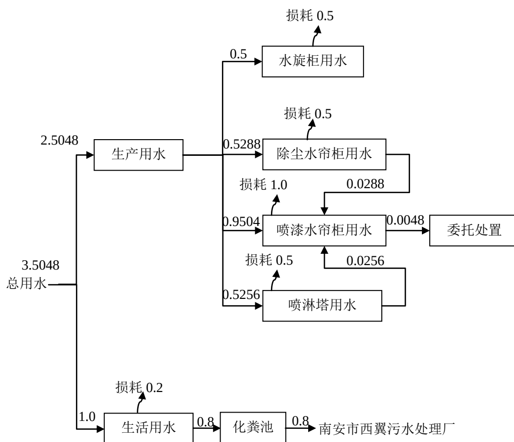
图 2.6-1 项目水平衡图 单位: t/d
