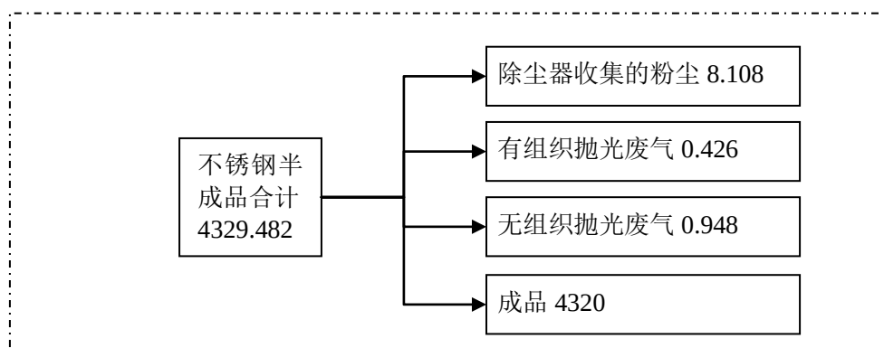
图 2.7-1 项目物料平衡图 (单位: t/a)
