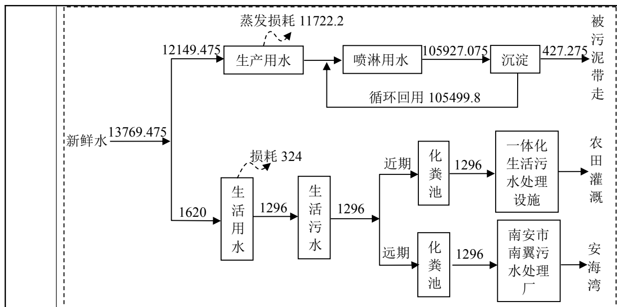
图 2-1 项目水平衡图（单位：m³/a）
